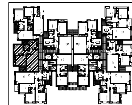
PLAN 4EME ETAGE
