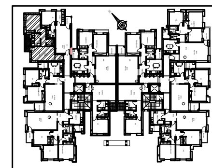
PLAN 1ER ETAGE
