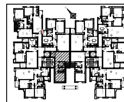
PLAN 1ER ETAGE
